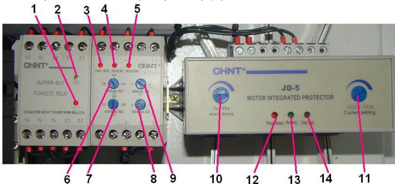
Рис.3 — Органы индикации и настройки реле шкафа управления.
