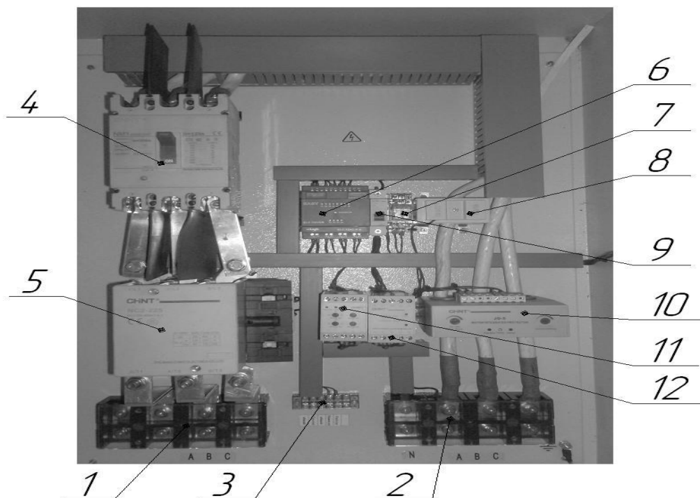
Рис. 1 — Размещение оборудования внутри шкафа станции.
