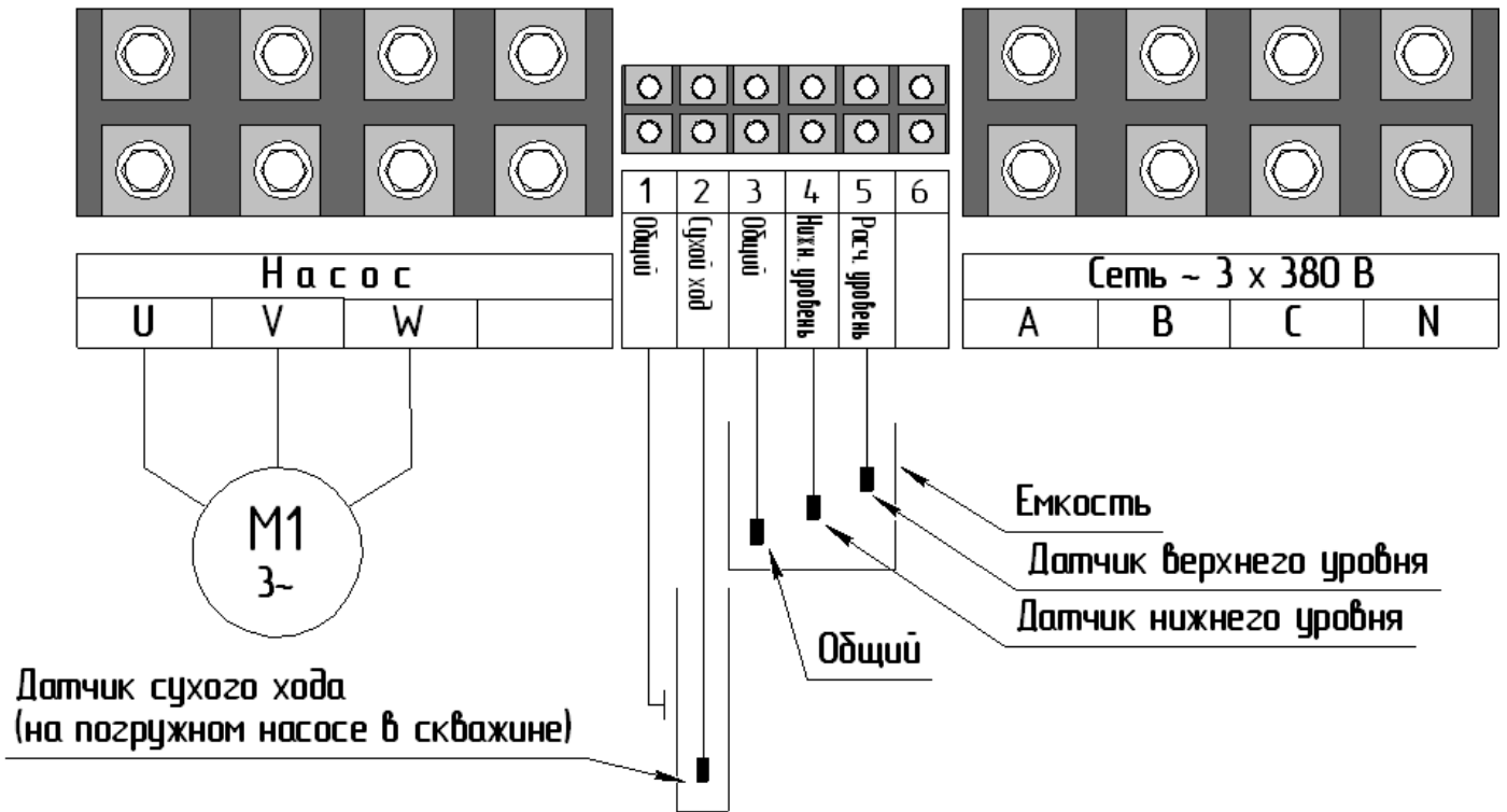
Рис. 4 — Обозначение клемм станции.
