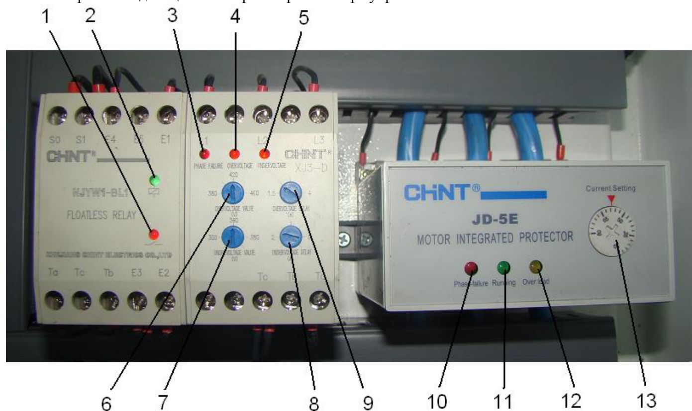
Рис.3 — Органы индикации и настройки реле шкафа управления.
