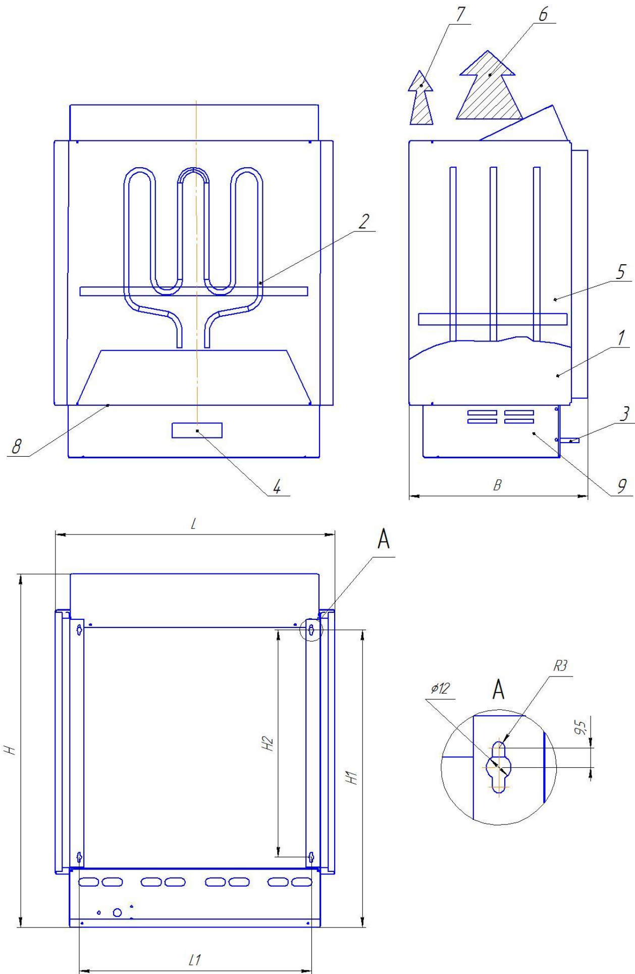
Рис.1 Электрокаменка серии ЭК. Устройство и габаритные размеры.
