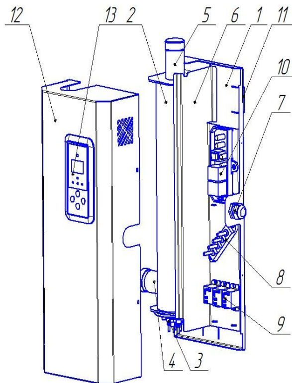
Сурет 1. Электр сужылытқыштың құрылысы
