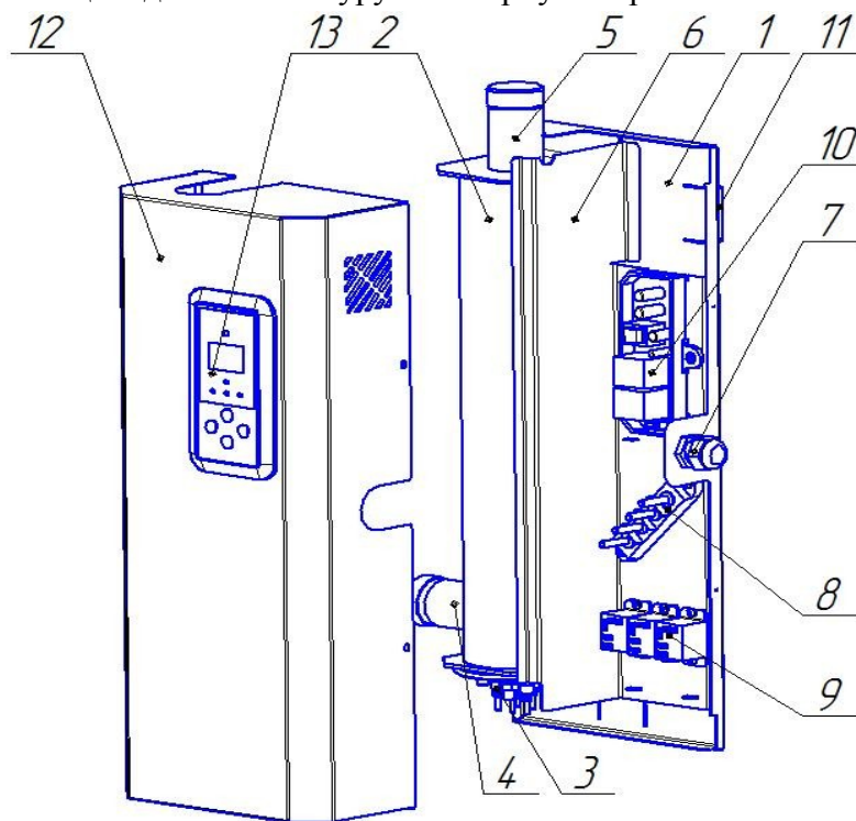
Рис.1 Конструкция электроводонагревателя
