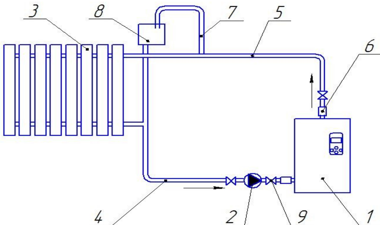
Сурет 4. Жылыту жүйесінде ЭСЖ пайдалану нұсқасы
