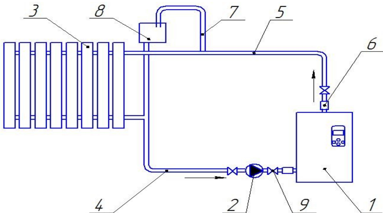
Сурет 4. Жылыту жүйесінде ЭСЖ пайдалану нұсқасы жарлығай) күйінде қосу ТҮЙІМ САЛЫНАДЫ!
