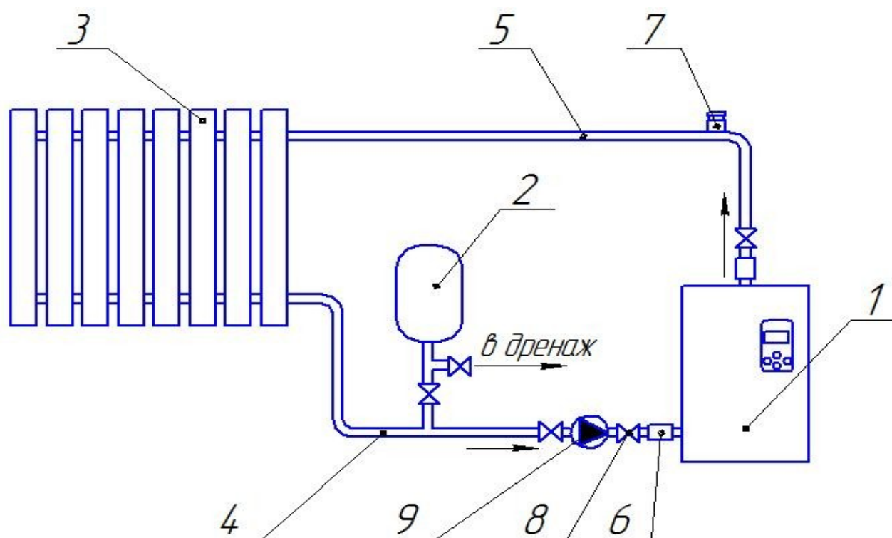
Сурет 5. Жылыту жүйесінде ЭСЖ пайдалану нұсқасы
